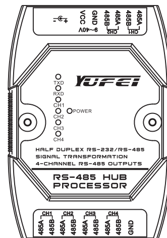
图1 YF-504CK-2顶部面板示意图
